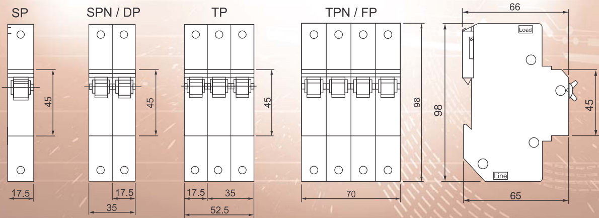
MCB 80A
